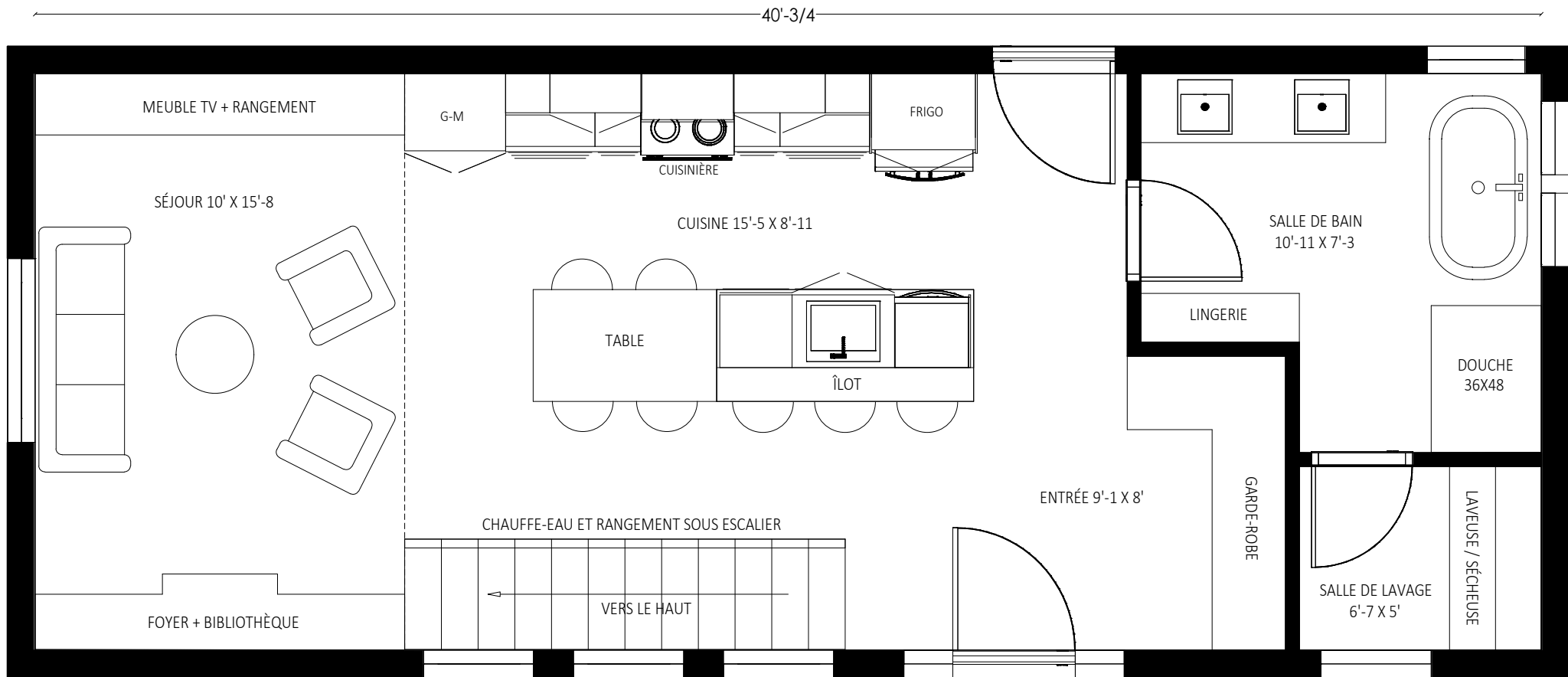
MODÈLE MEZZANINE 800 PC. REZ-DE-CHAUSSEZ
